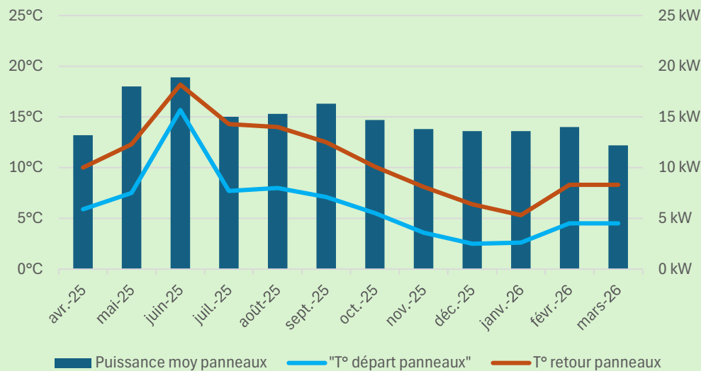
Fonctionnement des panneaux géothermiques
